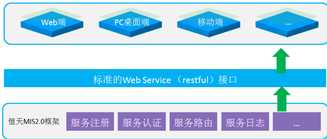
图一：恒天 MIS 2.0 框架
